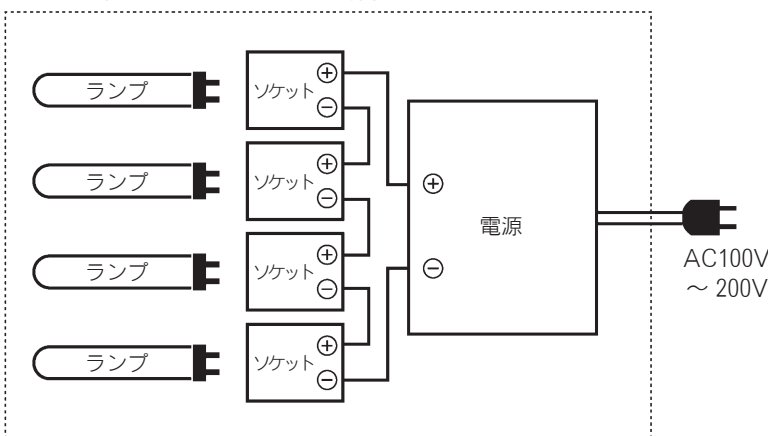
最終接続図 (ランプ4灯の場合)
