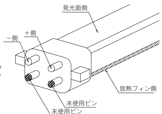
蛍光灯型LEDランプのピン配置
